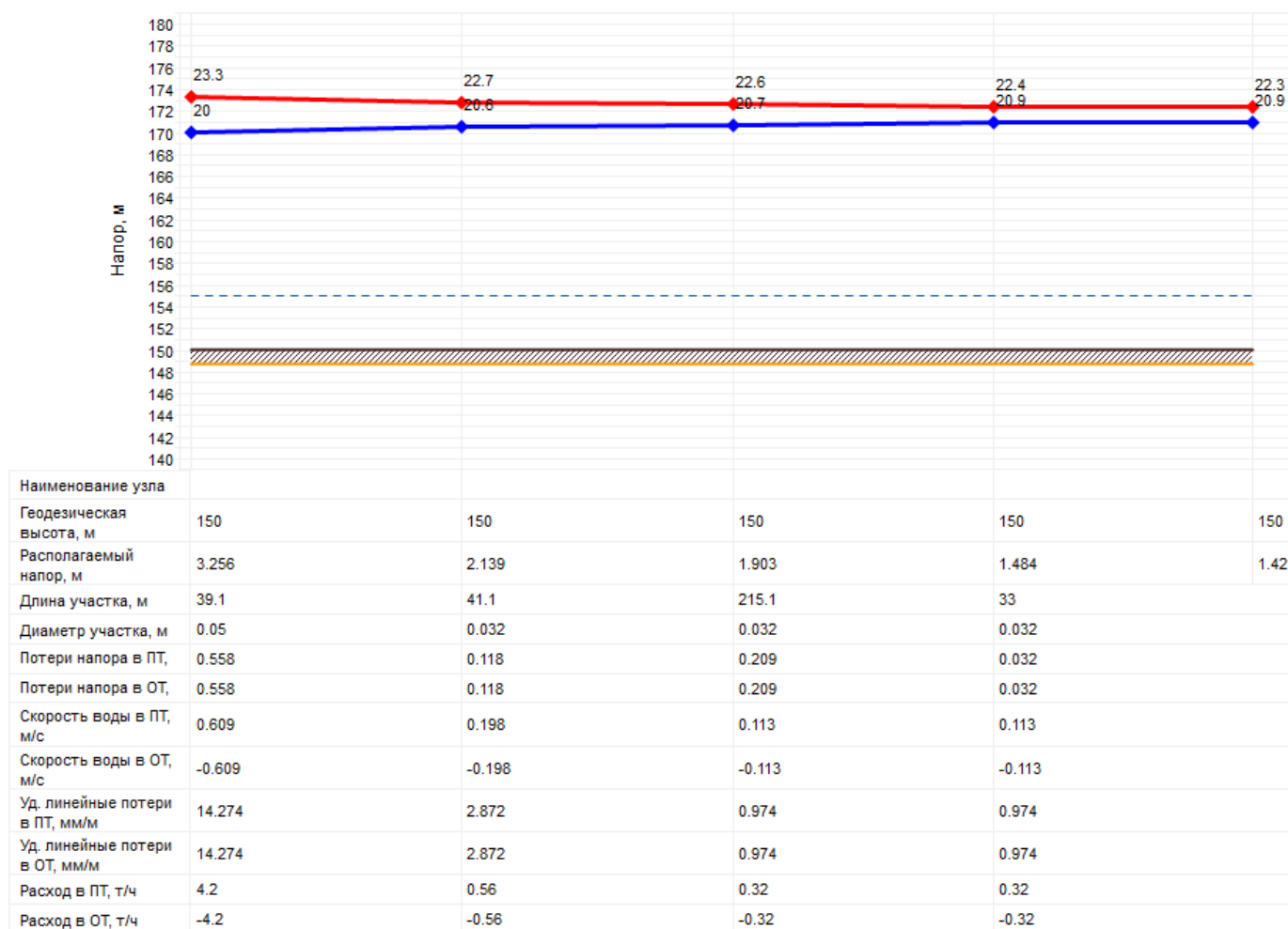
Рисунок 2.4 – Пьезометрический график тепловой сети котельной с. Буготак
