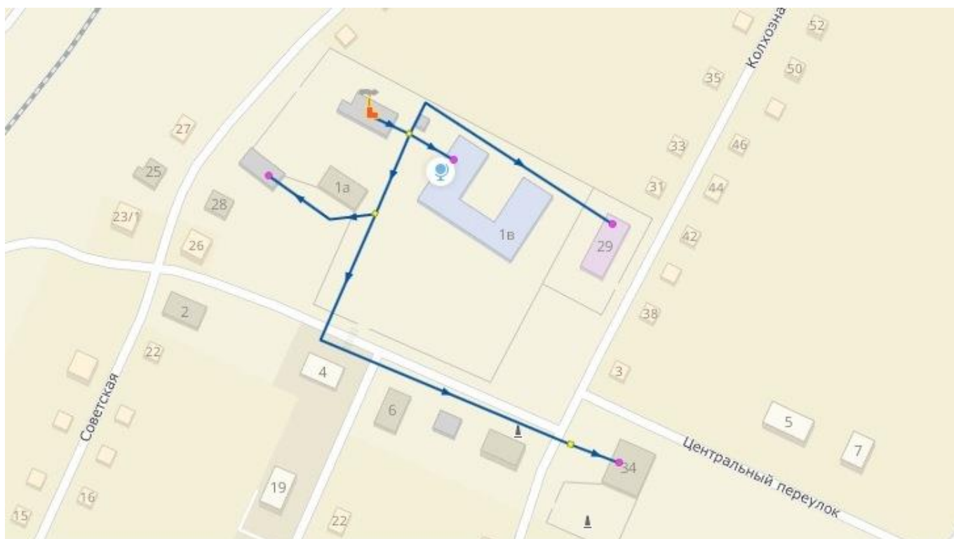
Рисунок 2.5 – Модель системы теплоснабжения котельной с. Буготак
