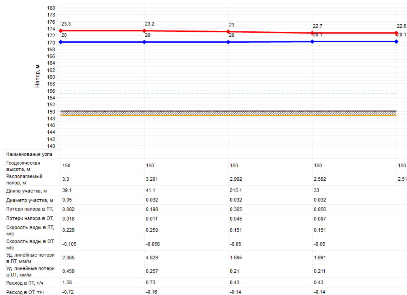
Рисунок 2.9 – Пьезометрический график от источника теплоснабжения (котельной с. Буготак) до самого удаленного потребителя
