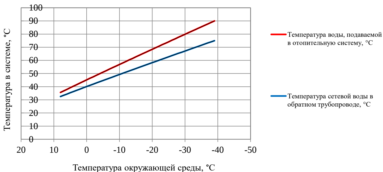
Рисунок 2.3 – График изменения температур теплоносителя 90–75 °С
