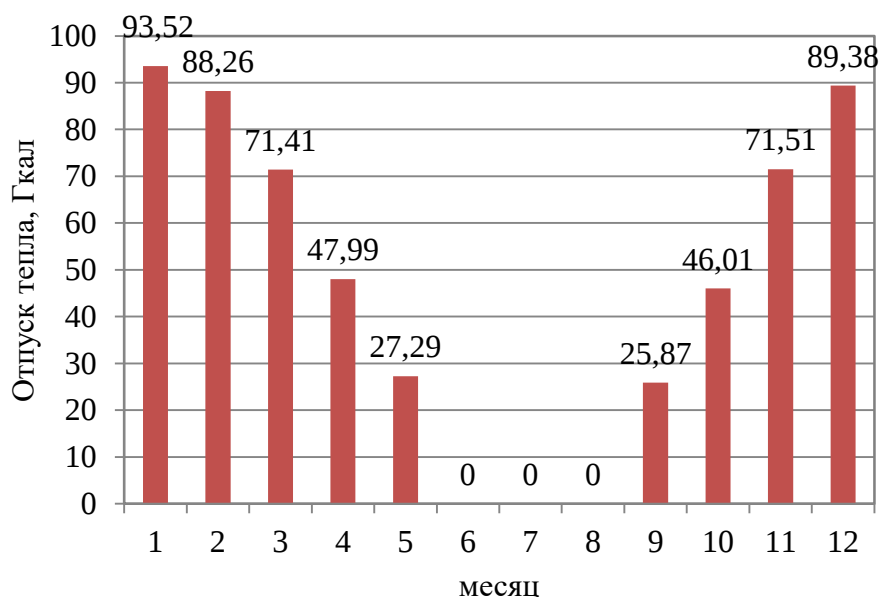
Рисунок 1.7 – Оптимальный температурный график отпуска тепловой энергии для котельной с. Буготак
