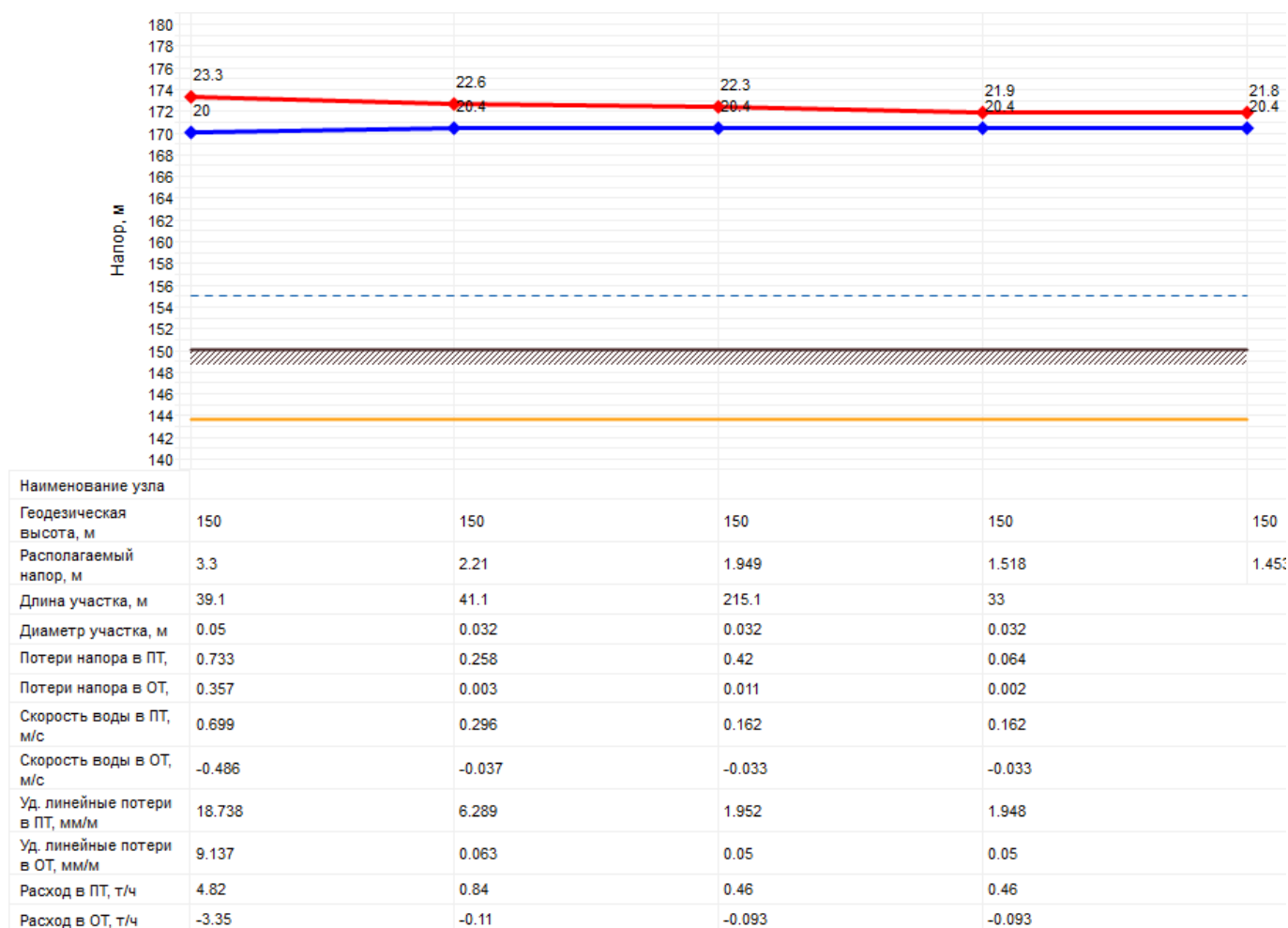
Рисунок 2.10 – Пьезометрический график от источника теплоснабжения (котельной с. Буготак) до самого удаленного потребителя
