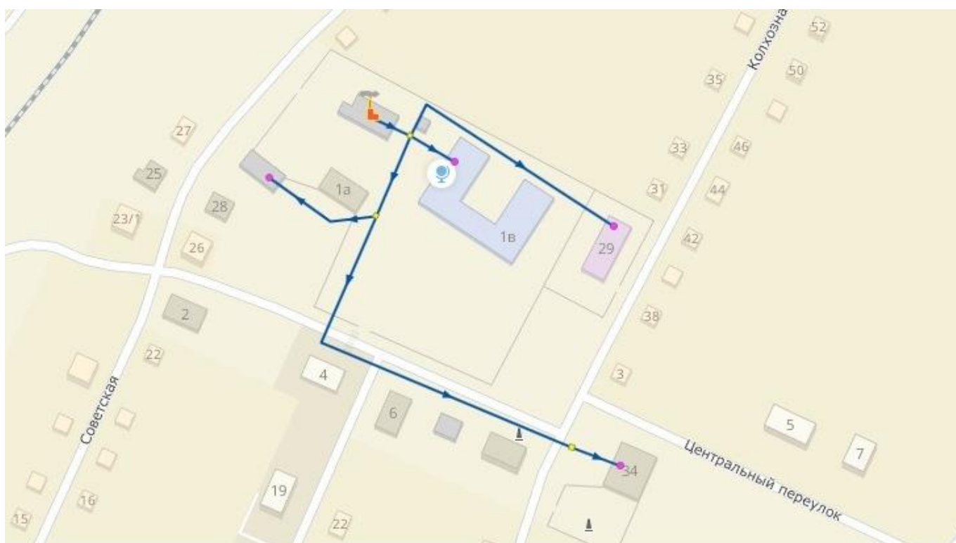
Рисунок 2.8 – Модель системы теплоснабжения котельной с. Буготак
